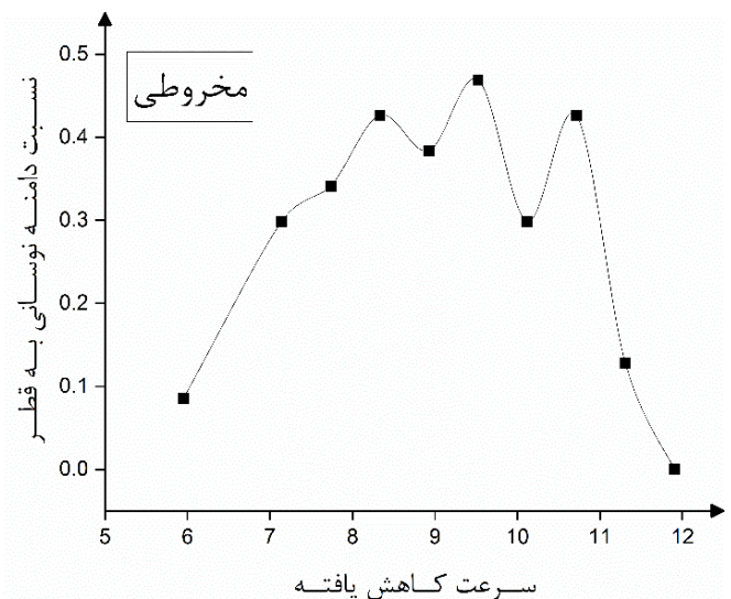
شکل ۱۳: نمودار دامنه نوسانی ایجاد شده بی بعد بر حسب سرعت کاهش یافته برای آزمایش استوانه مخروطی
