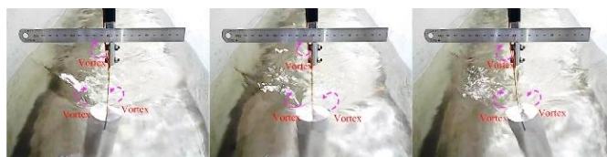
شکل ۶: تصاویر دوربین از VIV یک استوانه دایروی [4]
