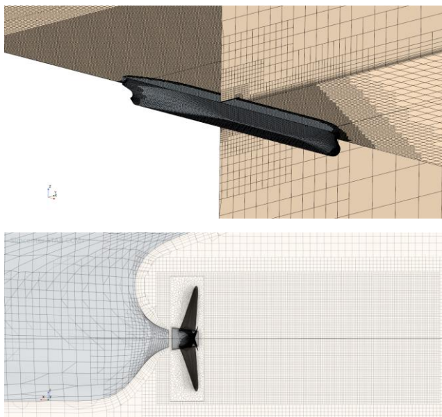
شکل ۵- نمای کلی از مش اطراف بدنه و پروانه.
