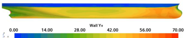
شکل ۶- توزیع مقدار y^+ بر روی بدنه.
