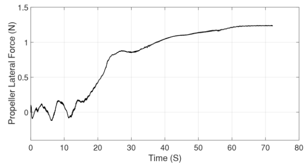
شکل ۱۶: نیروی عرضی ایجاد شده توسط پروانه در مانور توقف در عدد فرود ۰/۰۹۸۱
