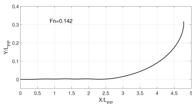
شکل ۱۳- مسیر توقف کشتی در عدد فرود ۰/۱۴۲
