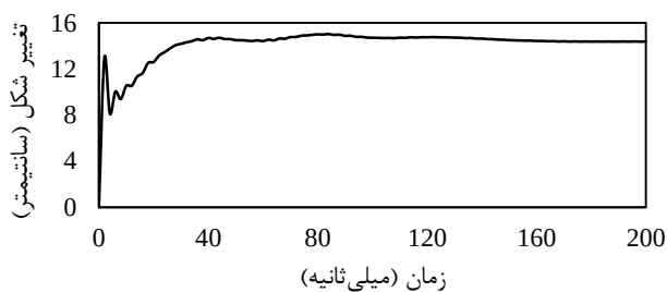
شکل ۱۰ - تغییر شکل نزدیک‌ترین نقطه به مرکز انفجار بر روی شمع
