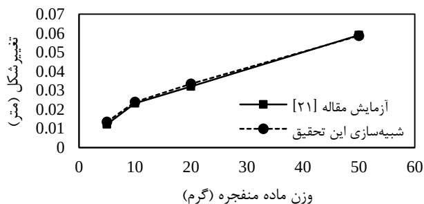
شکل ۵ - مقایسه تغییر شکل مرکز صفحه در آزمایش مرجع [۲۱] و شبیه‌سازی این تحقیق
