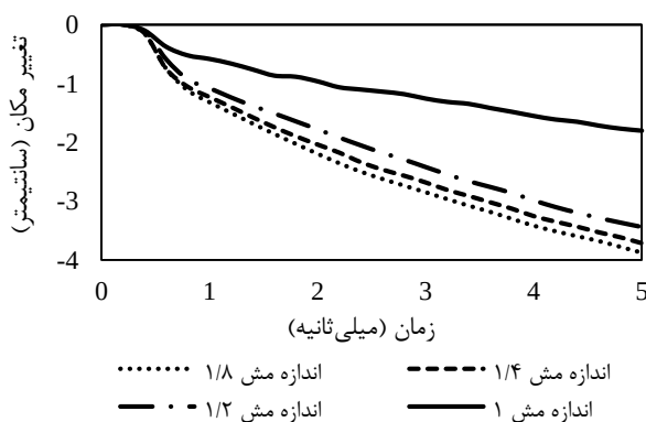
شکل ۹ - مقایسه تاثیر تغییر اندازه شبکه کل نمونه مدل‌سازی بر تغییر مکان نزدیک‌ترین نقطه از شمع به مرکز انفجار (کاهش اندازه شبکه به نسبت‌های ۰،۵، ۰،۲۵ و ۰،۱۲۵)
