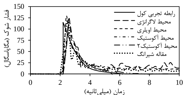
شکل ۳ - مقایسه تاریخچه زمانی فشار ناشی از انفجار زیر آب در میدان آزاد برای رابطه تجربی، مقاله و شبیه‌سازی‌های این تحقیق
