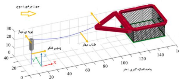
شکل ۵- قفس کشتی مانند تک مهاره [۲۶].
