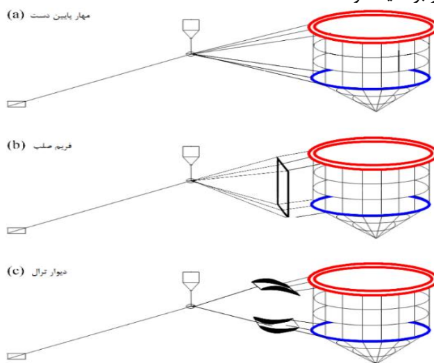
شکل ۴- انواع اقدامات جهت افزایش استحکام در سیستم قفس تک مهار [۷].
