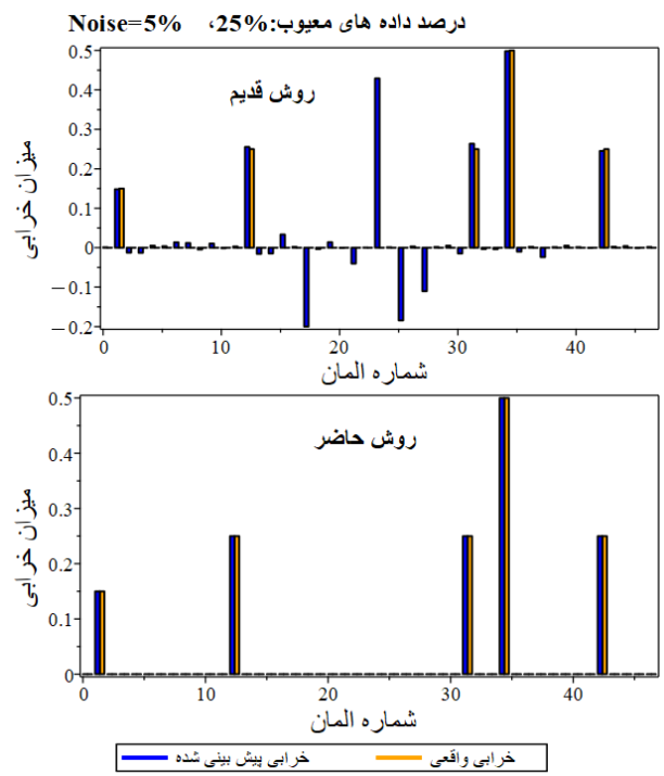
شکل ۶: مقایسه نتایج روش حاضر و روش مرسوم برای حالت خرابی ۶ المان با داده‌های نویزدار.
