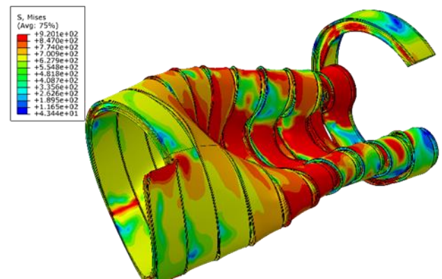
شکل ۱۶ لایه کارکس مدل بیونیک تحت فشار ۵۲/۲ مگاپاسکال
