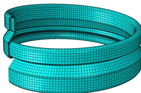
شکل ۶ نمودار همگرایی مش و مش‌بندی حلقه کارکس
