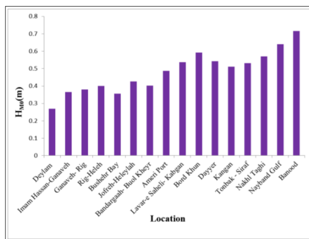
شکل ۶-الف- مقدار متوسط ارتفاع موج در هر ایستگاه
