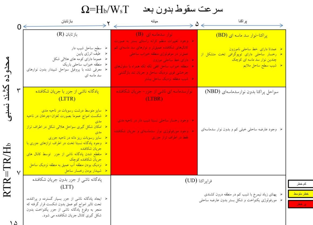
شکل ۴- مدل وضعیت ساحل - حالت ساحل تابعی از سرعت سقوط بدون بعد ( \Omega ) و محدوده کشند نسبی (RTR) [۲۵ و ۲۰]
