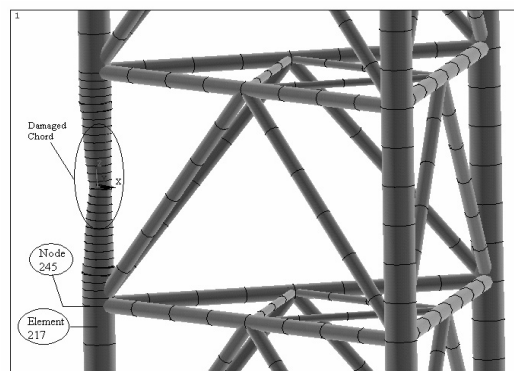
شکل ۱۰- نمایی از وتر صدمه دیده در برخورد از پهلوی کشتی
