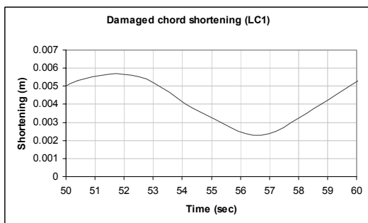
شکل ۲۴- میزان کوتاه شدگی وتر ضربه خورده در حالت صدمه دیده در طی پریود ششم
