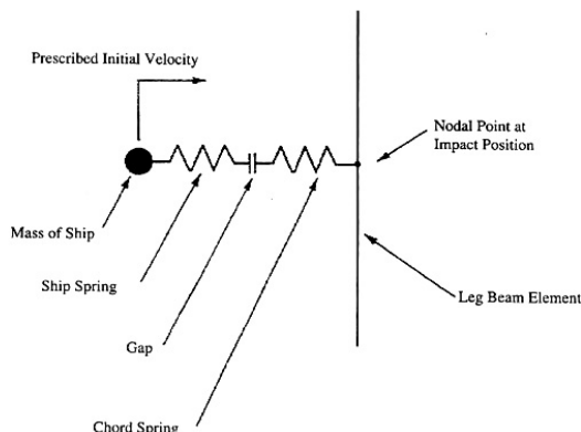
شکل ۴- روش مدل‌سازی دینامیکی تصادم کشتی و سکو [۳]
