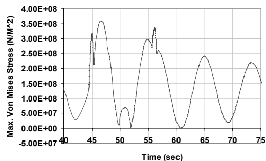
شکل ۲۱- تاریخچه زمانی تنش فون میسز Von Mises حداکثر برای عضو ضربه خورده در طی تصادم اولیه و ثانویه
