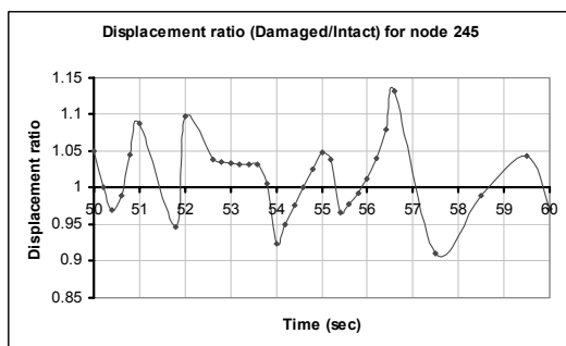
شکل ۲۳- مقایسه نسبت تغییرمکان گره ۲۴۵ در حالت سکوی صدمه دیده به سالم در طی پریود ششم
