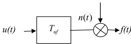
شکل ۱ - مدل خطی (SISO) برای معادله موریسون
