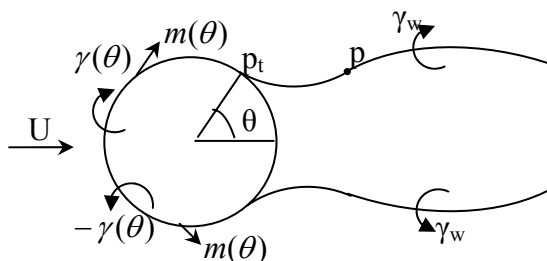
شکل ۲- توزیع سینگولاریته ها
