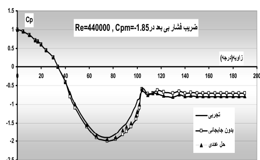
شکل ۵- توزیع فشار بی بعد برای رینولدز ۴۴۰۰۰
