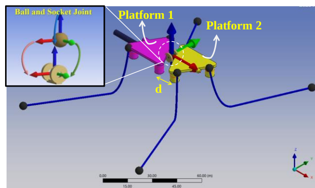
شکل ۵- دو پلتفرم همراه با اتصال بال جوینت و سیستم مهار
