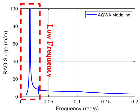
شکل ۶- عملکرد دامنه پاسخ حرکت سرج با در نظر گرفتن سیستم مهار
