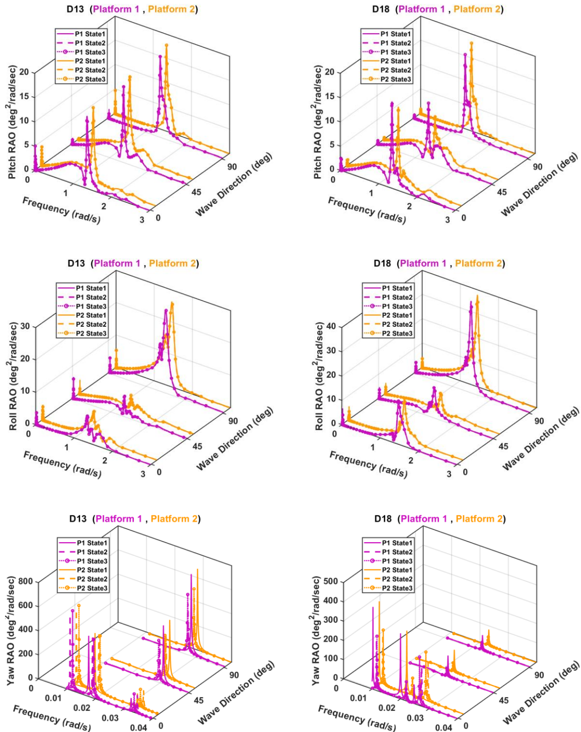
شکل ۸- منحنی RAO پلتفرم‌های خورشیدی برای حرکات Pitch, Roll, Yaw در فاصله D13, D18 در سه جهت موج ۴۵ و ۹۰ درجه
