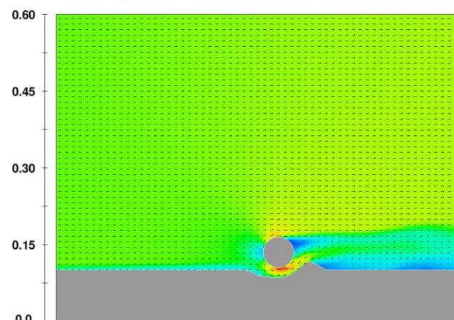
شکل ۶- پروفیل آبستگی برای t=50 s
