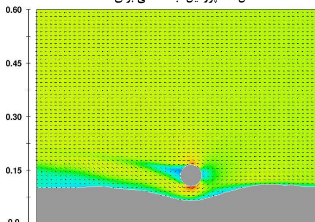
شکل ۱۳- پروفیل آبستگی برای t=2400 s (سیکل سوم)
