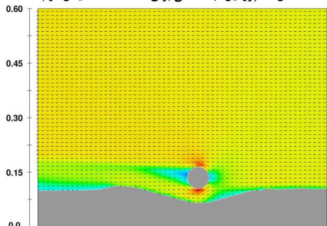
شکل ۱۱- پروفیل آبستگی برای t=1600 s
