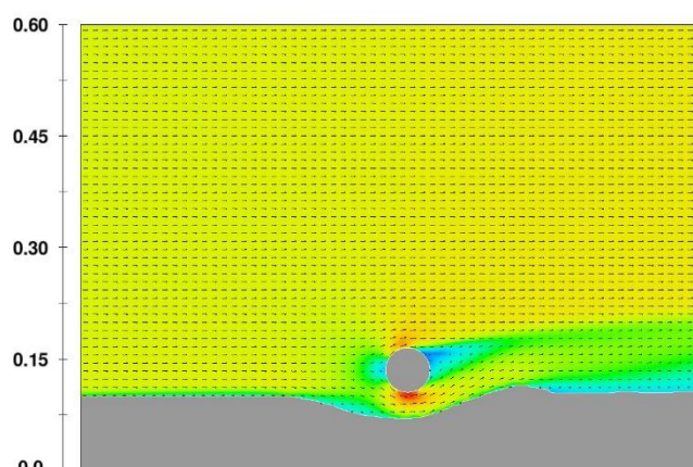
شکل ۱۰- پروفیل آبستگی برای t=1200 s (سیکل دوم)
