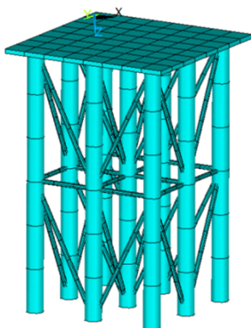
شکل ۲- شبکه‌بندی متناظر مدل فیزیکی و مدل عددی تهیه شده در نرم‌افزار ANSYS
