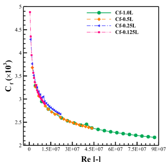
شکل ۷ - نمودار ضریب مقاومت اصطکاکی بر حسب عدد رینولدز در مقیاس‌های متفاوت
