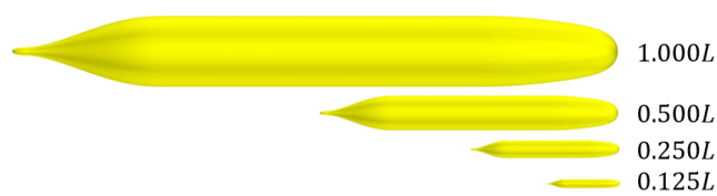
شکل ۲- ابعاد مختلف شناور های مقیاس شده
