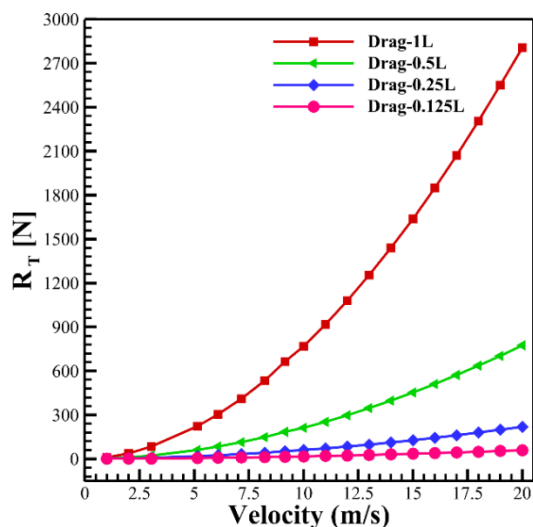
شکل ۸ - نمودار ضریب مقاومت کل بر حسب عدد سرعت
