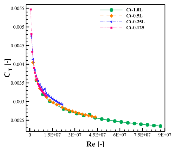
شکل ۶ - نمودار مقادیر مقاومت و ضریب مقاومت کل بر حسب عدد رینولدز
