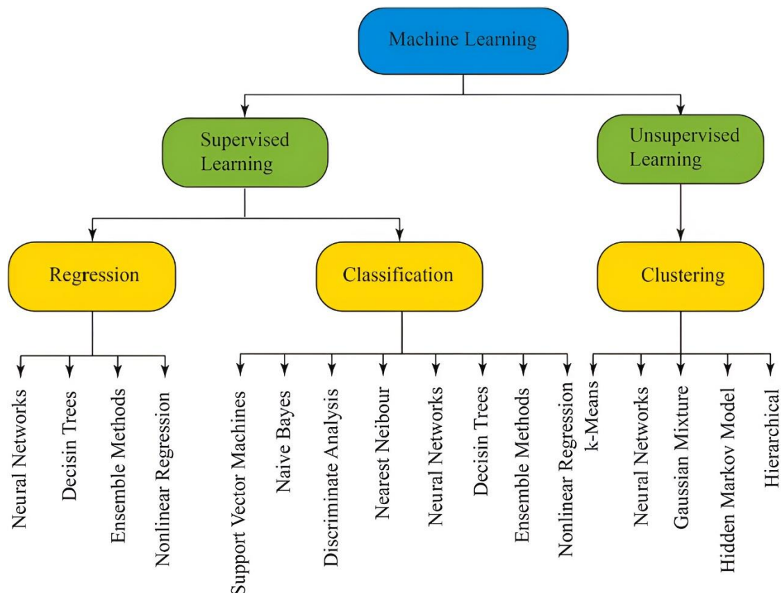
شکل ۳- الگوریتم‌های رایج یادگیری ماشین مورد استفاده در کاربردهای مهندسی [۱۶]
