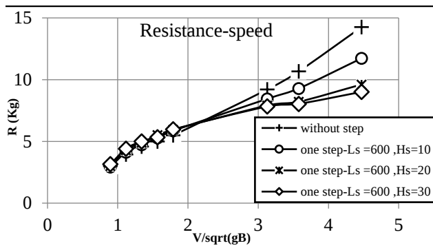
شکل ۸- تغییر ارتفاع پله در فاصله ۰/۲۴ طول کلی از ترانسوم و ددرايز ۲۰ درجه
