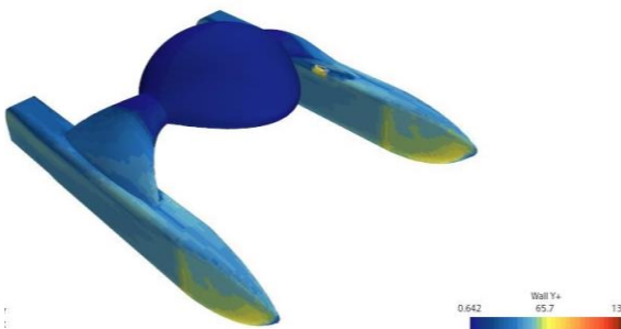
شکل ۸ - نمایی از مقادیر Y^+ بر روی بدنه شناور در سرعت 3 \text{ m/s}
