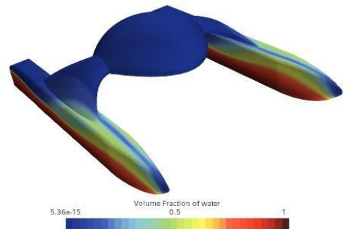
شکل ۲۰- نمایی از بالا آمدن آب بر روی بدنه در سرعت ۳ m/s
