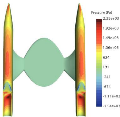
شکل ۲۲ - نمایی از فشار وارده بر روی شناور با وزن ۲۴ kg
