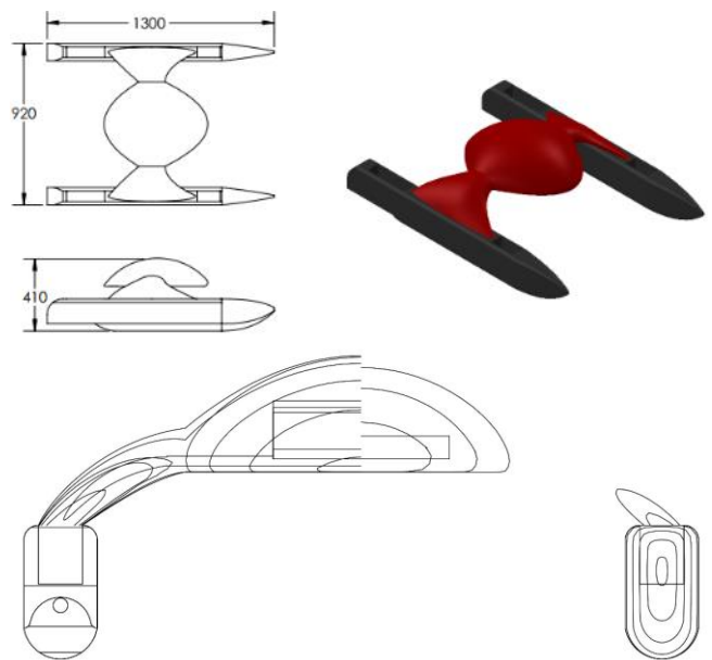
شکل ۱ - نمایی از هندسه و خطوط بدنه شناور آرین
