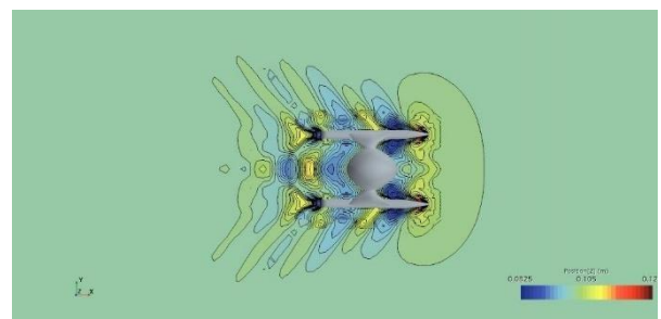
شکل ۱۰ - نمایی از سطح آزاد در سرعت 1 \text{ m/s}
