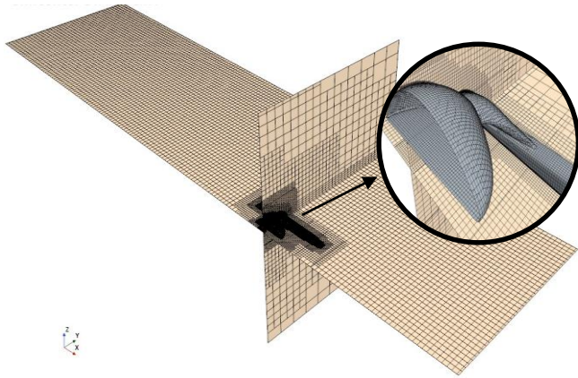
شکل ۲ - نمایی از دامنه محاسباتی
