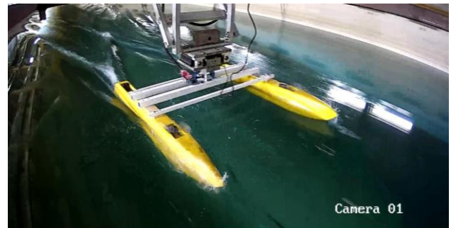
شکل ۱۷ - نمایی از تست مدل با وزن ۲۰ kg در سرعت ۳ m/s
