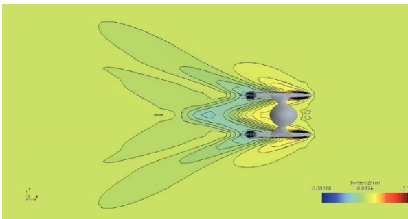
شکل ۱۳ - نمایی از سطح آزاد در سرعت 3 \text{ m/s}
