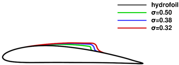
شکل ۲۷ - مقایسه شکل حباب تشکیل شده با افزایش عدد کایتاسیون هیدروفویل ناکا ۴۴۱۲ در زاویه حمله ۲/۵ درجه و عمق غرق شدگی ۰/۵ طول وتر هیدروفویل
