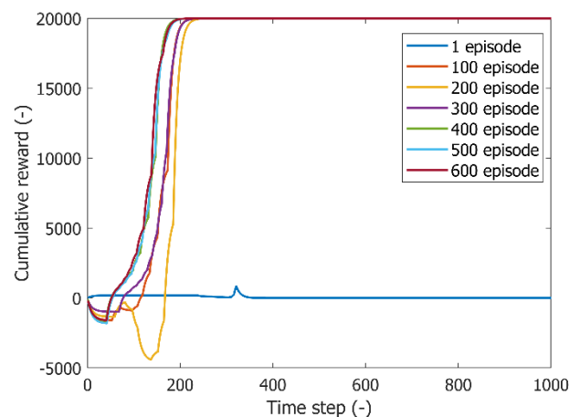
شکل ۴- پاداش‌های انباشته شده براساس تعداد اپیزود تعقیب عمق ۱ متر
