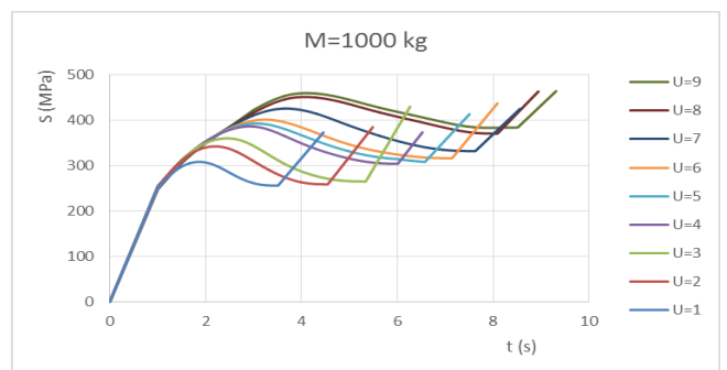
شکل ۸- رشد تنش در زمان برخورد لنگر ۱ تنی با لوله
