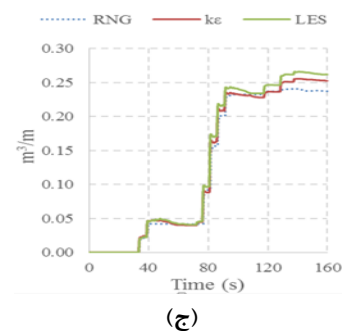
شکل ۳- نتایج حساسیت سنجی مدل عددی نسبت به مدل‌های آشفتگی (الف) سطح آزاد (ب) فشار دینامیکی (ج) روگذری
