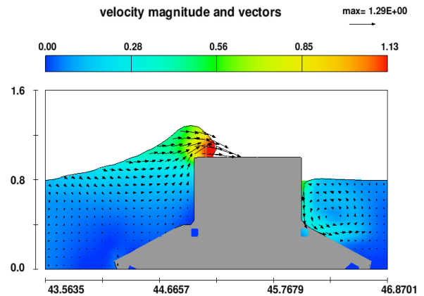
میدان سرعت موج برای موج شکن کیسونی
