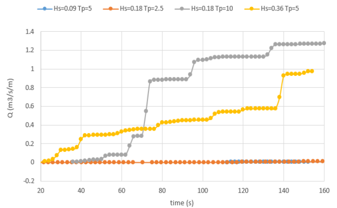
شکل ۱۲- اثر مشخصات موج در مقدار روگذری موج از موج‌شکن کیسونی حفره‌دار نوع دو
