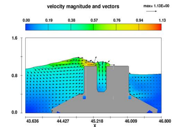
میدان سرعت موج برای موج شکن کیسونی حفره دار- نوع اول
