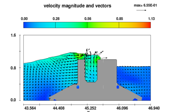
میدان سرعت موج برای موج شکن کیسونی حفره دار- نوع دوم
