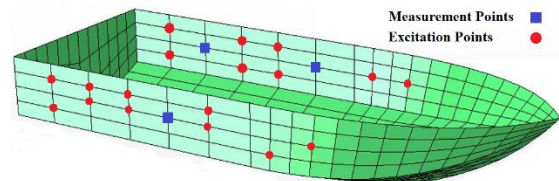
شکل ۱۰. نقاط تحریک و اندازه‌گیری مدل پوسته بدنه شناور
