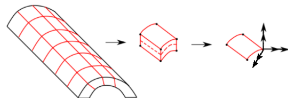
شکل ۵. نمایش شماتیک جزء پوسته چهار گره‌ای
