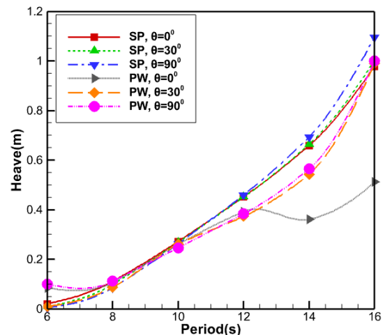
شکل ۲۳- تاثیر زاویه برخورد موج روی دامنه هیو سکوی ترکیبی و سکوی تنها
