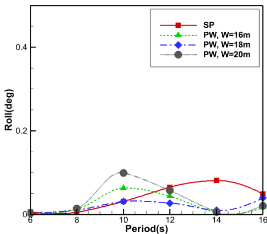
شکل ۱۲- تاثیر پهنای فلپ روی دامنه رول سکوی ترکیبی و سکوی تنها
