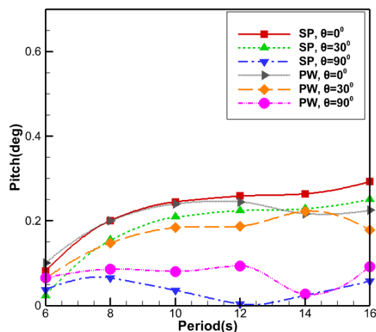
شکل ۲۵- تاثیر زاویه برخورد موج روی دامنه پیچ سکوی ترکیبی و سکوی تنها
