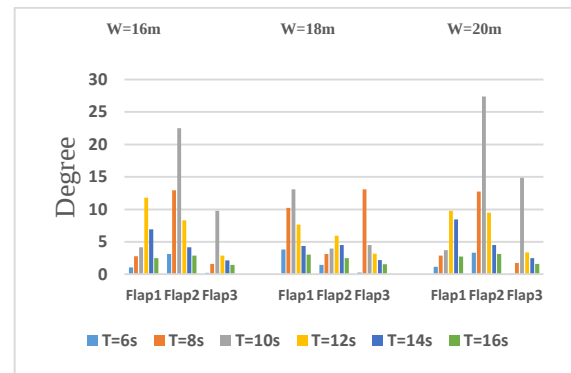
شکل ۱۴- تاثیر پهنای فلپ روی دامنه جابجایی فلپ‌ها
