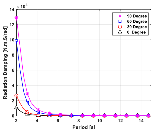
شکل ۲۲- ضریب میرایی تشعشعی برای فلپ در حالت های مختلف چیدمان زاویه ای ماژول ها
