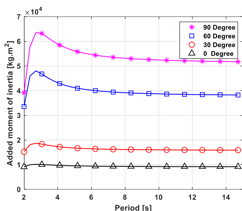
شکل ۲۱- ضریب ممان اینرسی جرمی افزوده برای فلپ در حالت های مختلف چیدمان زاویه ای ماژول ها
