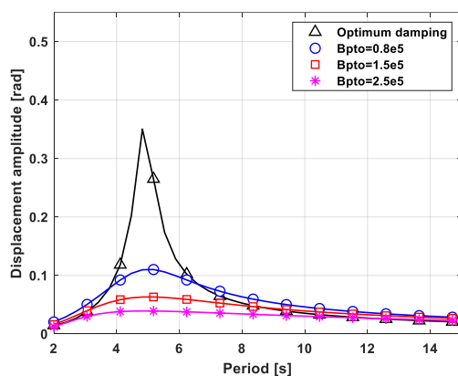
شکل ۶- مقایسه جابجایی زاویه‌ای فلپ با دو استراتژی میرایی ثابت و میرایی بهینه برای PTO
