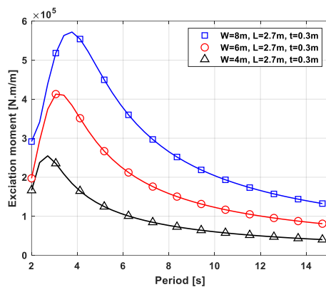
شکل ۱۱- ممان تحریک بر حسب پریود برای سه پهنای مختلف
