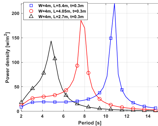
شکل ۱۶- چگالی سطحی توان تولیدی بر حسب پریود برای سه ارتفاع مختلف فلپ
