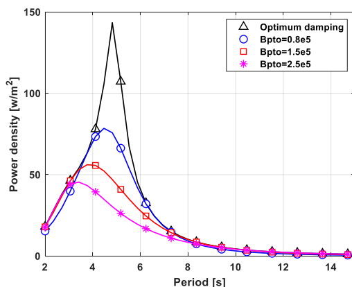
شکل ۷- مقایسه چگالی سطحی توان تولیدی با دو استراتژی میرایی ثابت و میرایی بهینه برای PTO
