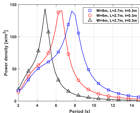
شکل ۱۳- چگالی سطحی توان تولیدی بر حسب پریود برای سه پهنای مختلف
