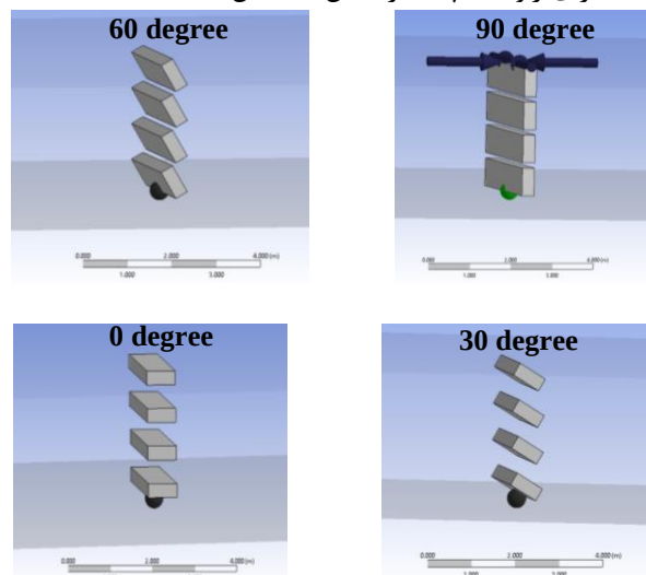
شکل ۲۰- مبدل انرژی ماژوله شده با جهت گیری مختلف ماژول ها
