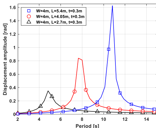
شکل ۱۵- دامنه جابجایی زاویه‌ای بر حسب پیوند برای سه ارتفاع مختلف فلپ
