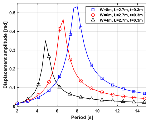
شکل ۱۲- دامنه جابجایی بر حسب پریود برای سه پهنای مختلف
