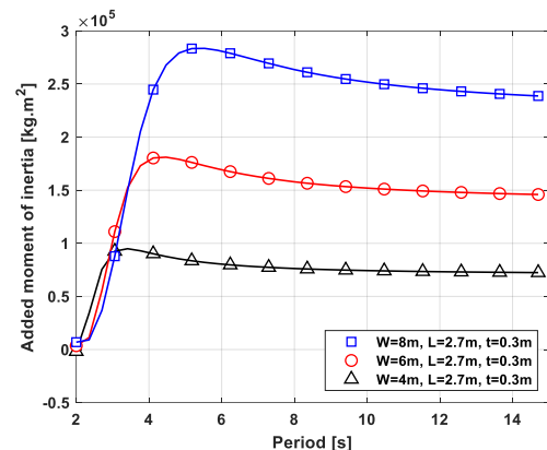
شکل ۹- ممان اینرسی افزوده بر حسب پریود برای سه پهنای مختلف
