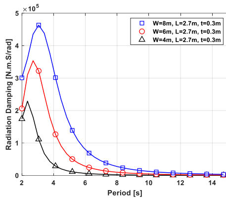
شکل ۱۰- میرایی تشعشعی بر حسب پریود در سه پهنای مختلف
