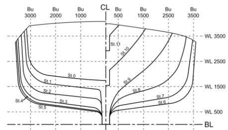
شکل ۲- نقشه خطوط بدنه لنج
