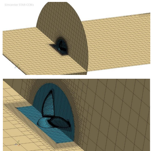
شکل ۱۵- شبکه بندی دامنه حل اطراف پروانه
