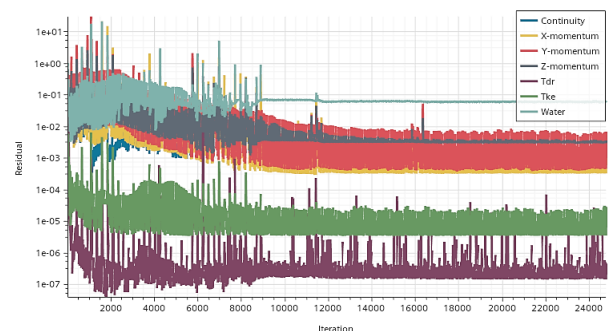
شکل ۷ - تاریخچه همگرایی و مقادیر باقیمانده معادلات حاکم
