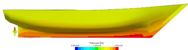
شکل ۲۴- توزیع فشار روی بدنه لنج در سرعت نهایی
