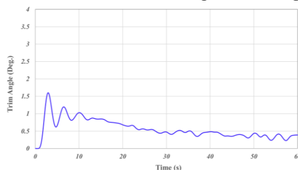
شکل ۲۶- تغییرات زاویه تریم بدنه لنج بر حسب زمان
