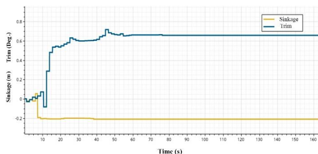
شکل ۱۱- تغییرات تریم و سینکیج بدنه لنج در سرعت ۵/۱۴ m/s
