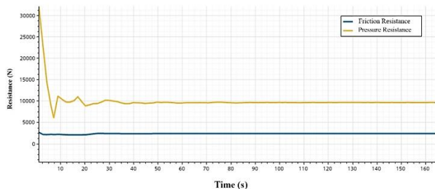
شکل ۱۲- تغییرات مولفه های مقاومت لنج در سرعت ۵/۱۴ m/s
