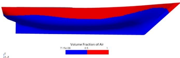
شکل ۹ - کانتور کسر حجمی سیال روی بدنه لنج در سرعت ۵/۱۴ m/s
