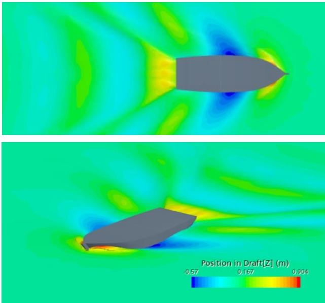
شکل ۸ - امواج تولید شده اطراف بدنه لنج در سرعت ۵/۱۴ m/s
