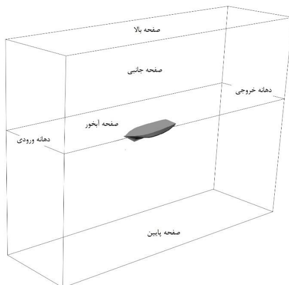
شکل ۴ - دامنه محاسباتی استفاده شده در مدلسازی عددی
