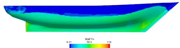
شکل ۶ - مقدار Y^+ بر روی بدنه لنج
