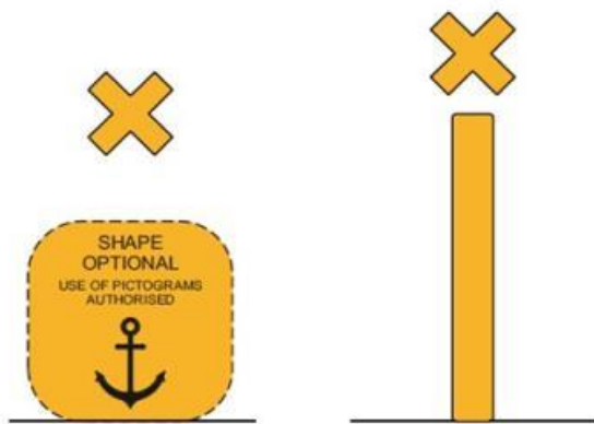
شکل ۸- بویه‌های علائم ویژه
