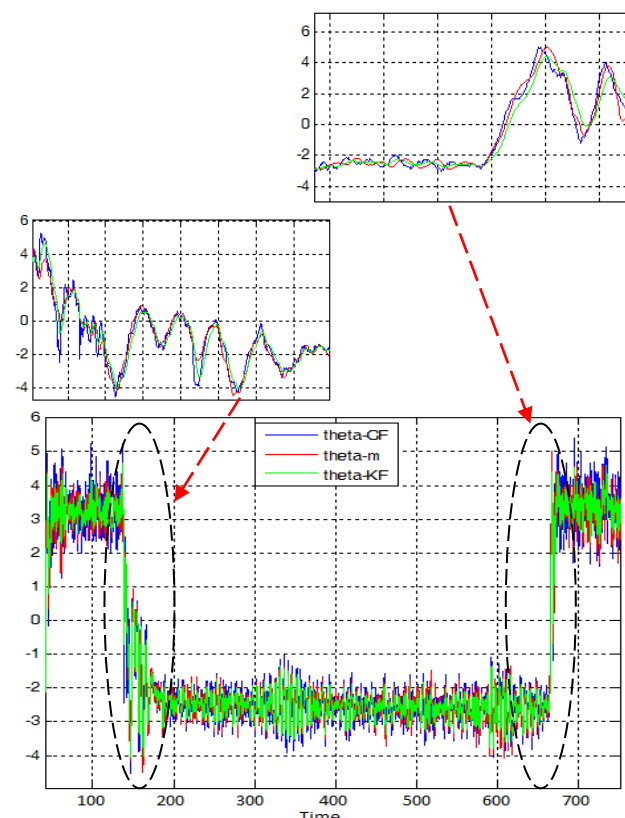
شکل ۷- زاویه فراز اندازه گیری شده و تخمین زاویه فراز با فیلتر CF تطبیقی و کالمن (درجه)
