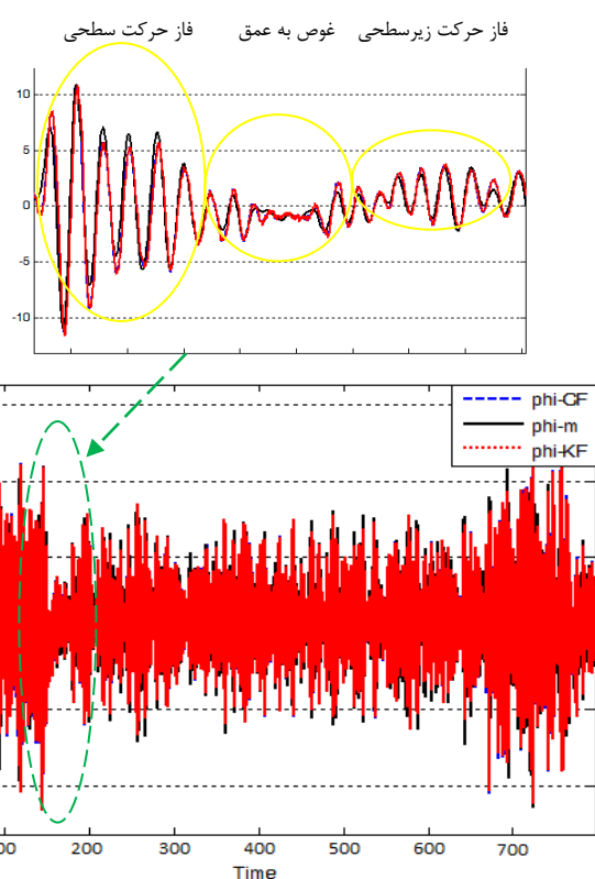
شکل ۶- مقدار واقعی زاویه غلتش و مقدار تخمینی با فیلتر مکمل تطبیقی و فیلتر کالمن (درجه)
