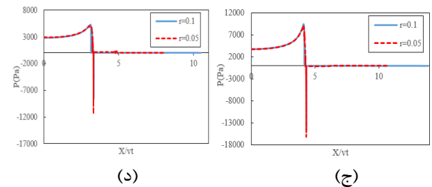
شکل ۱۱. نمودار توزیع فشار در شعاع ۰/۱ و ۰/۰۵ در قسمت قبل از تونل برای زوایای خیز کف: (الف) ۱۰ درجه، (ب) ۱۵ درجه، (ج) ۲۰ درجه و (د) ۲۵ درجه.
