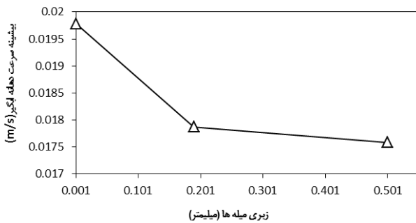
شکل ۶ - تغییرات بیشینه سرعت جریان در دهانه آبنگهی برای میله هایی با زبری (میلی متر) A: 0.001 ، B: 0.19 و C: 0.5
