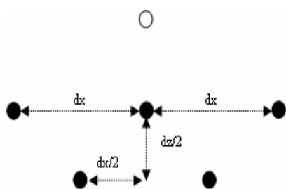
شکل ۱- نحوه قرارگیری ذرات مرزی در شرط مرزی دینامیکی (دوایر توخالی و توپر، به ترتیب نمایانگر ذره سیال و ذرات مرزی می‌باشند).
