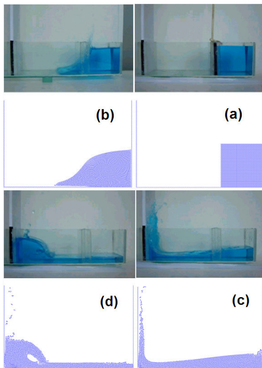
شکل ۵- مقایسه نتایج مدل عددی با نتایج آزمایشگاهی عیسی آزمایش شکست سد، در زمان‌های: a) t=0/0 b) t=0/16 c) t=0/485 و d) t=0/89 ثانیه
