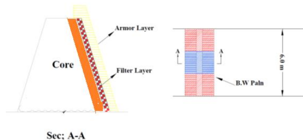
شکل ۵- پلان و نحوه چینش مصالح آرمور، فیلتر و هسته در فلوم آزمایشگاهی (بخش آبی: محل اجرا مدل فیزیکی)
