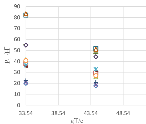
شکل ۱۵: نمودار بدون بعد تغییرات فشار خروجی در برابر دوره تناوب موج برای شیب قائم
