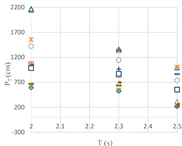
شکل ۱۴: تغییرات فشار خروجی در برابر دوره تناوب موج برای شیب قائم
