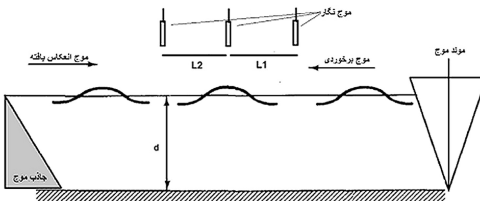
شکل ۵- نمای شماتیک از محل قرار گرفتن موج نگار در کانال موج ساز
