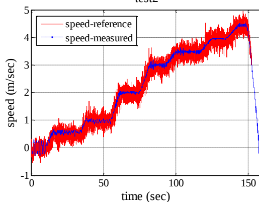
شکل (۶) خروجی سرعت مرجع و سرعت اندازه‌گیری شده توسط حسگر سرعت پیشنهادی در تست‌های ۱ و ۲.
