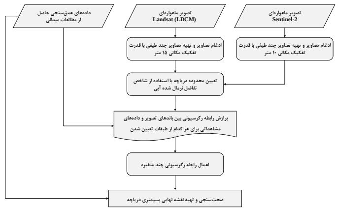
شکل ۴- فلوچارت نحوه استخراج نقشه عمق سنجی بر اساس داده‌های
