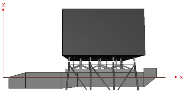
شکل ۲ - مدل شناور-سازه پشتیبیان-عرشه
