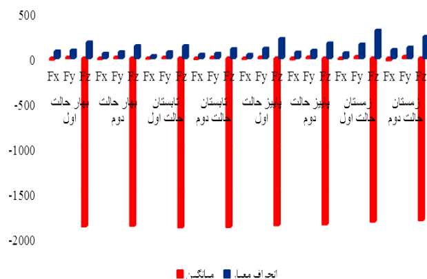
شکل ۱۱- میانگین و تغییرات نیروهای وارد بر المان های میتینگ
