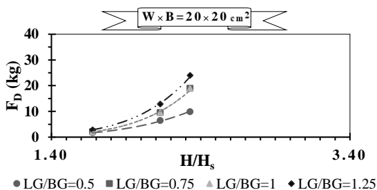
شکل ۵- نیرو کششی بر حسب نسبت ارتفاع موج قبل از پوشش به ارتفاع موج بعد از پوشش، در چیدمان مستطیلی با فواصل مختلف پوشش
