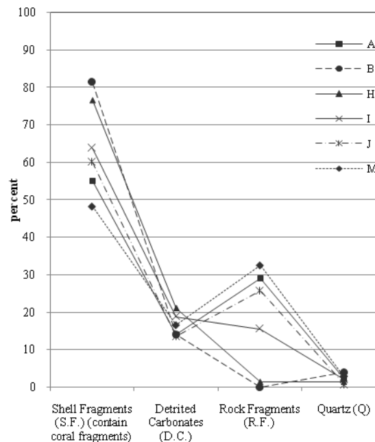
شکل ۱۱- درصد وزنی جنس ذرات رسوبی نمونه‌های A, B, H, I, J و M
