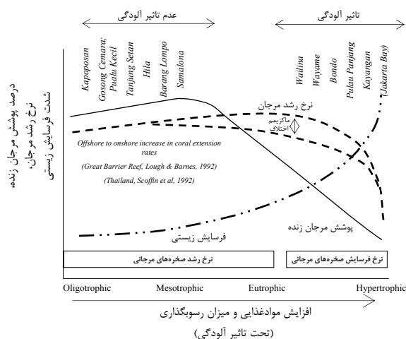
شکل ۸- خلاصه‌ای از عوامل موثر بر مرجانها [۱۴]
