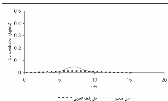
شکل ۱۳ - نمودار تغییرات غلظت در مکان (x و \delta ) در T=70 s
