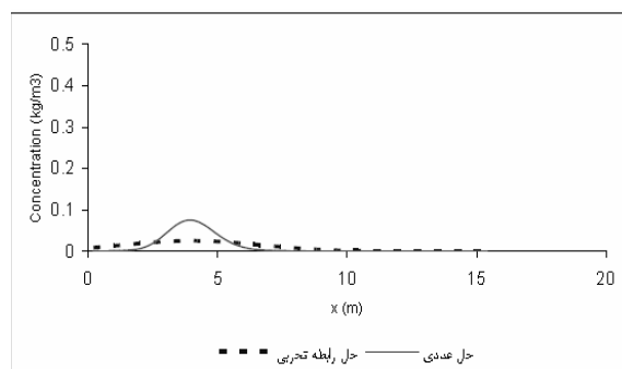
شکل ۱۲ - نمودار تغییرات غلظت در مکان (x و \delta ) در T=40 s
