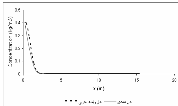
شکل ۱۰ - نمودار تغییرات غلظت در مکان (x و \delta ) در T=2.5 s [مبدا مختصات بر روی نقطه رها شده لکه نفتی قرار دارد]
