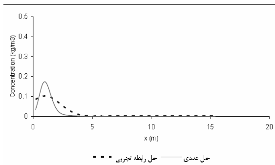
شکل ۱۱ - نمودار تغییرات غلظت در مکان (x و \delta ) در T=10 s
