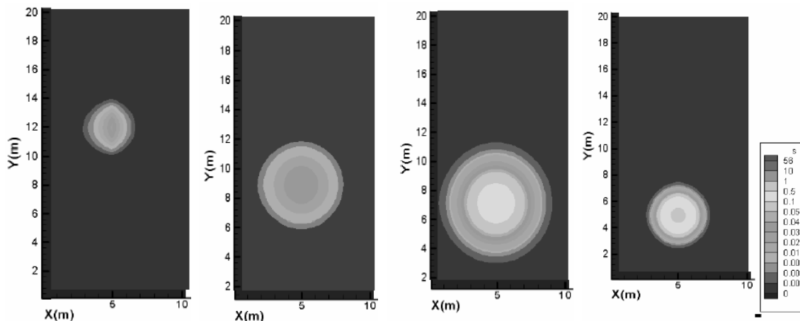
شکل ۶ - تغییرات غلظت نفت در ستون آب، T=2.5 s [ s بر حسب kg/m^3 ]
