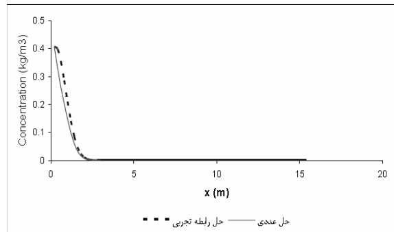
شکل ۱۰ - نمودار تغییرات غلظت در مکان (۵ و x) در T=2.5 s [مبدا مختصات بر روی نقطه رها شده لکه نفتی قرار دارد]
