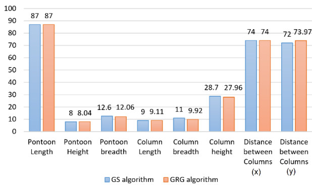
شکل ۶- مقایسه نتایج الگوریتم جستجوی شبکه‌ای با الگوریتم GRG
