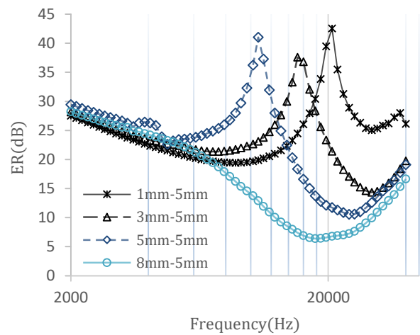
شکل ۲۰- نمودار ضریب کاهش اکو برای حفره های استوانه ای با قطر های متفاوت در لاستیک به ضخامت ۴۰ میلی متر
