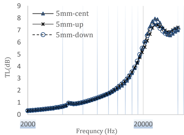
شکل ۱۷- اثر مکان قرار گیری حفره های استوانه‌ای بر روی ضریب افت انتقال در لایه لاستیک به ضخامت ۴۰ میلی متر
