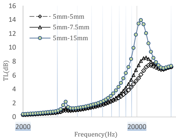
شکل ۲۱- اثر تغییرات طول استوانه به قطر ۵ میلی متر بر روی ضریب اتلاف انتقال در لایه لاستیک به قطر ۴۰ میلی متر
