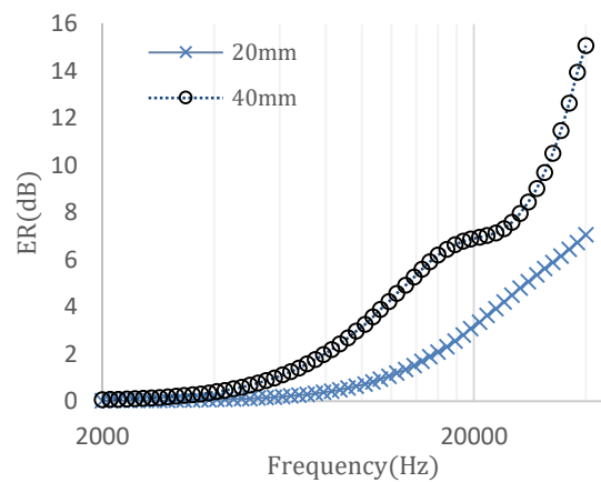
شکل ۹- تغییرات کاهش اکو در دو ضخامت مختلف در حالتی که محیط آکوستیک دو طرف مدل، هوا باشد
