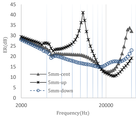
شکل ۱۸- اثر مکان قرار گیری حفره های استوانه‌ای بر روی ضریب کاهش اکو در لاستیک به ضخامت ۴۰ میلی متر
