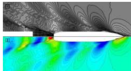
شکل ۱۳- الگوی موج کشتی KCS در آب آرام،
