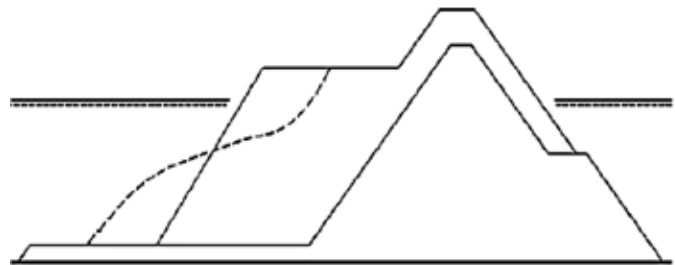
شکل ۱-ج- موج‌شکن سکویی همگن نسبتاً شکل‌پذیر
