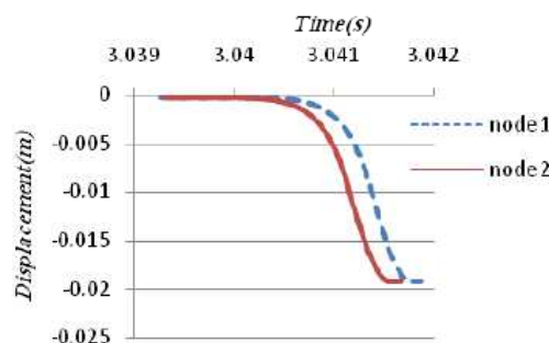
شکل ۷- نمودار تاریخچه زمانی جابجائی برای دو گره انتخابی روی مدل
