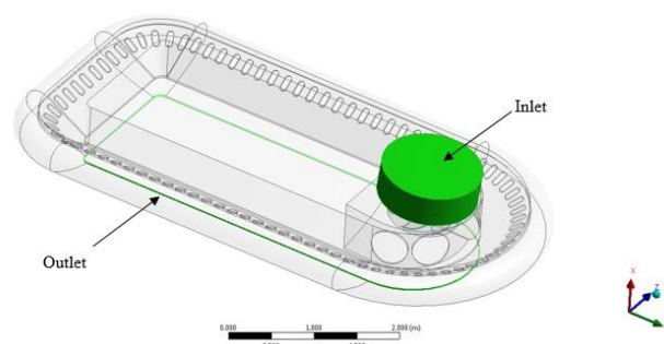
شکل ۷- ورودی و خروجی هاورکرافت
