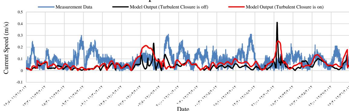
شکل ۲- سرعت جریان سطحی اندازه گیری شده (خط آبی رنگ)، جریان به دست آمده از اجرای مدل جریان در حالتی که ضرایب انتشار ثابت در نظر گرفته شدند (خط مشکی رنگ) و حالتی که مدول بستار تلاطم اعمال شده است (خط قرمز رنگ) در ایستگاه امیرآباد بین روزهای ۲۱ ماه نوامبر و ۳۱ ماه
