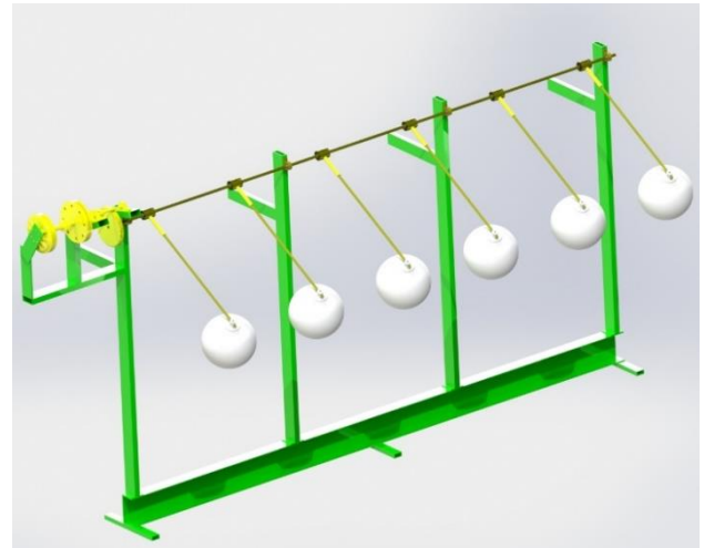
شکل ۴: سیستم مبدل انرژی موج طراحی شده از نوع سامانه ویواستار
