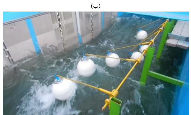
شکل ۸: (الف) موج منظم حاصل از سرعت ۲۵ rpm (ب) موج نامنظم حاصل از سرعت ۳۵ rpm
