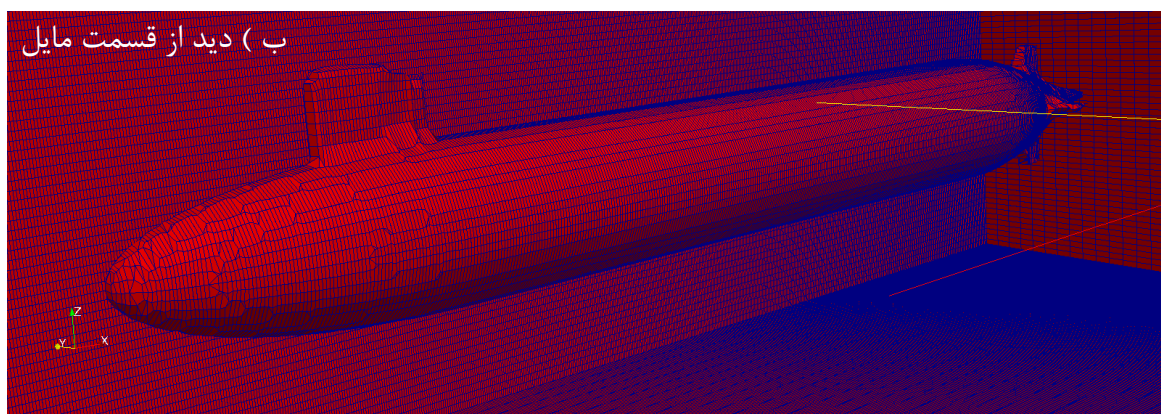
شکل ۶- فضای مش‌بندی اطراف متحرک Suboff 5470 (الف) دید از کنار (ب) دید از قسمت مایل
