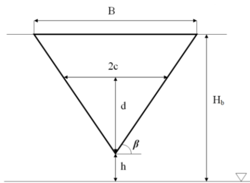
شکل ۲- مقطع گوه ای سینه شناور تندرو تک بدنه
