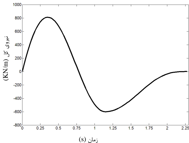
شکل ۷- نیروی گذرای کل اعمال شده بر سینه شناور مورد مطالعه در پدیده اسلمینگ
